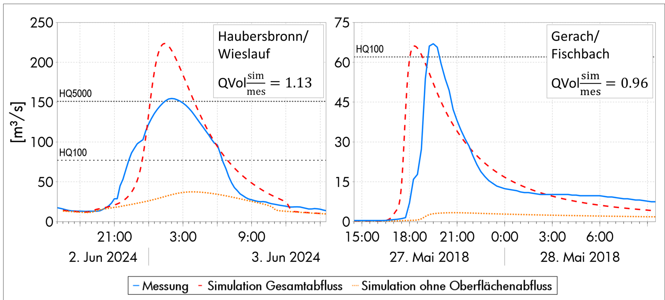
Ergebnisse mit LARSIM an den Pegeln
